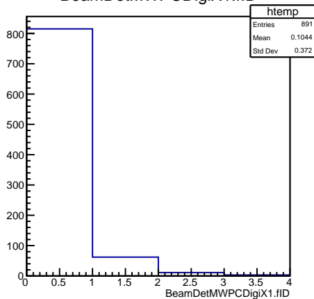
BeamDetMWPCDigiX1.fID
