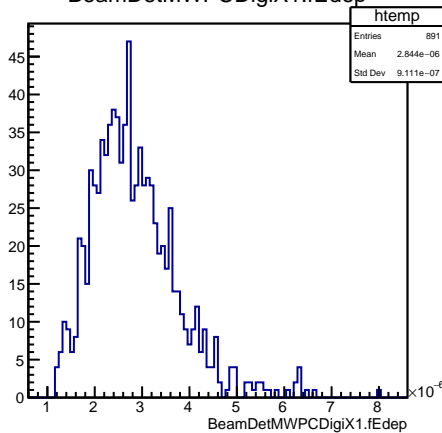
BeamDetMWPCDigiX1.fEdep
