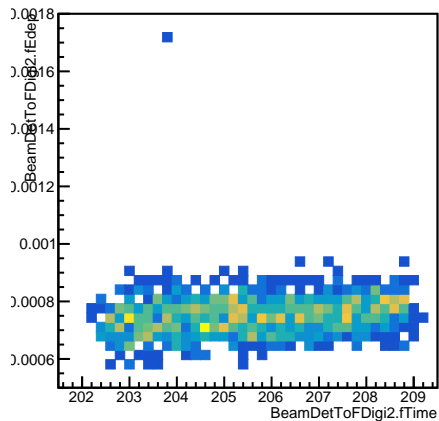
BeamDetToFdigi2.fTime (BeamDetToFdigi2.fdep&lt;0.016)
